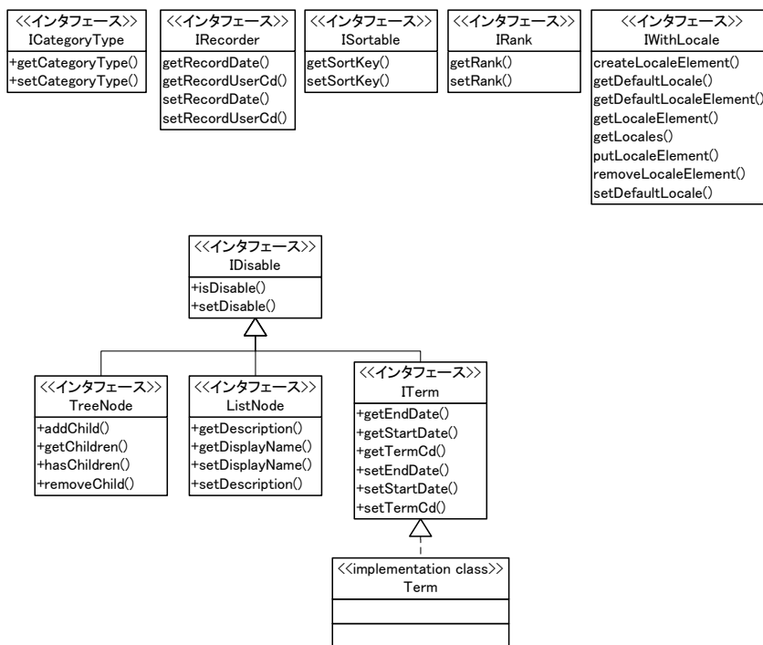
図 2-2 モデルクラスのインターフェース群
