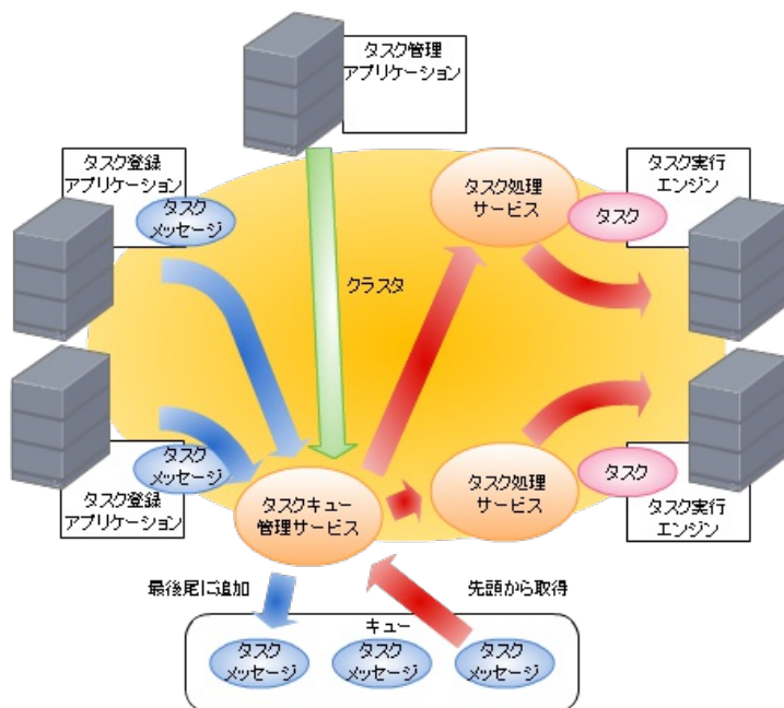
非同期処理機能の全体像（概要）
