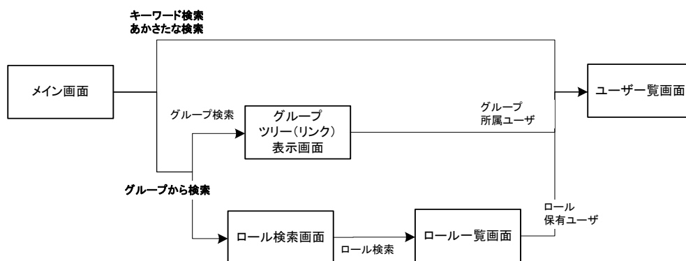
図 2-2 ユーザ検索の画面遷移
