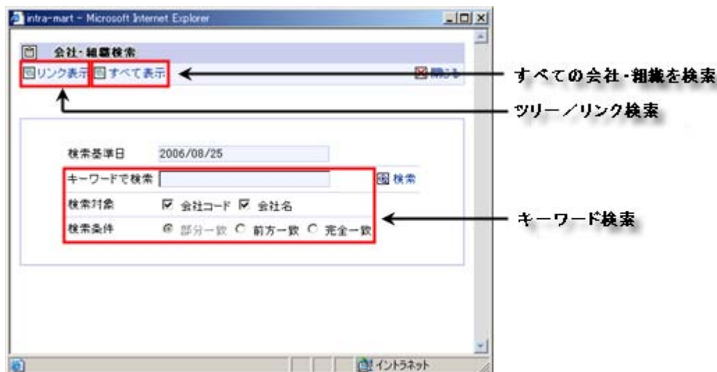
図 3-1 会社・組織検索のメイン画面
