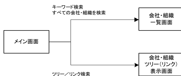
図 3-2 会社・組織検索の画面遷移
