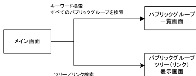
図 4-2 パブリックグループ検索の画面遷移
