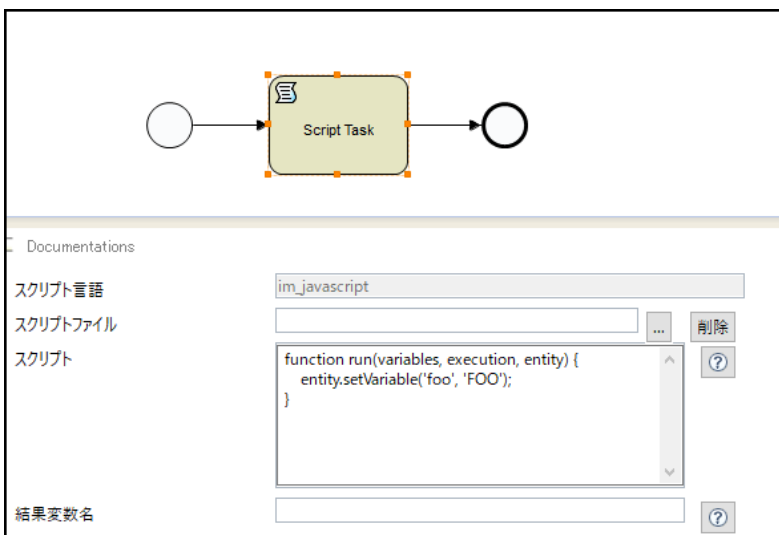
図：スクリプトタスク
