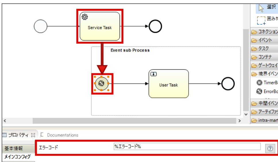
図：エラー開始イベント
