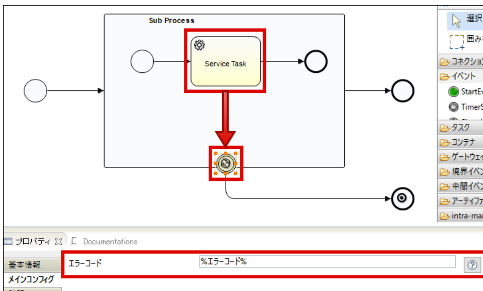
図：エラー境界イベント
