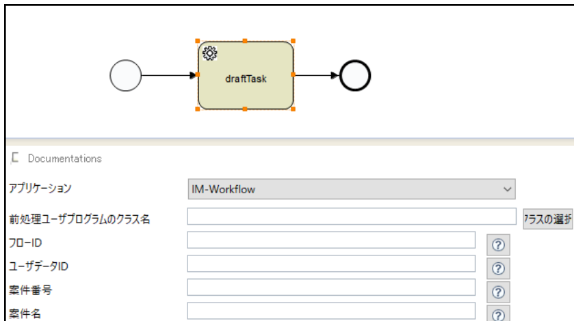
図：起票タスク
